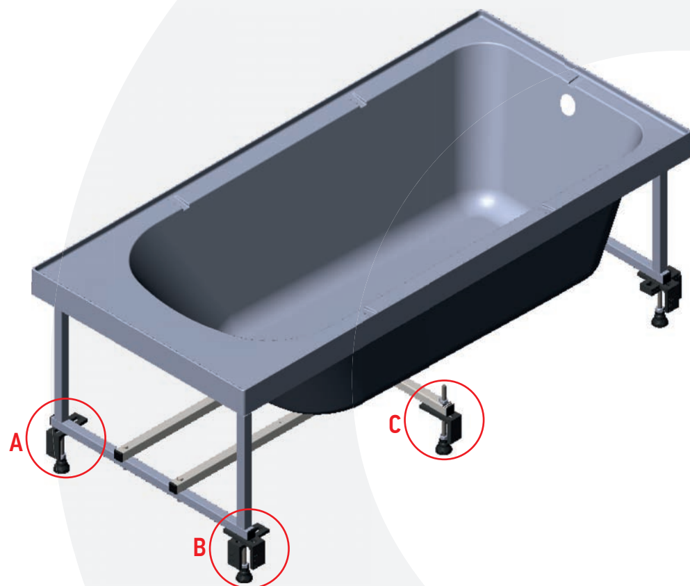
СБОРКА КАРКАСА ПОДДОНА БОКСОВ 1480x80
