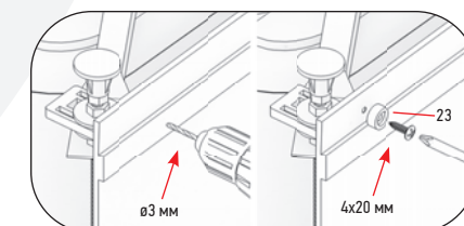
Установка экрана поддона
