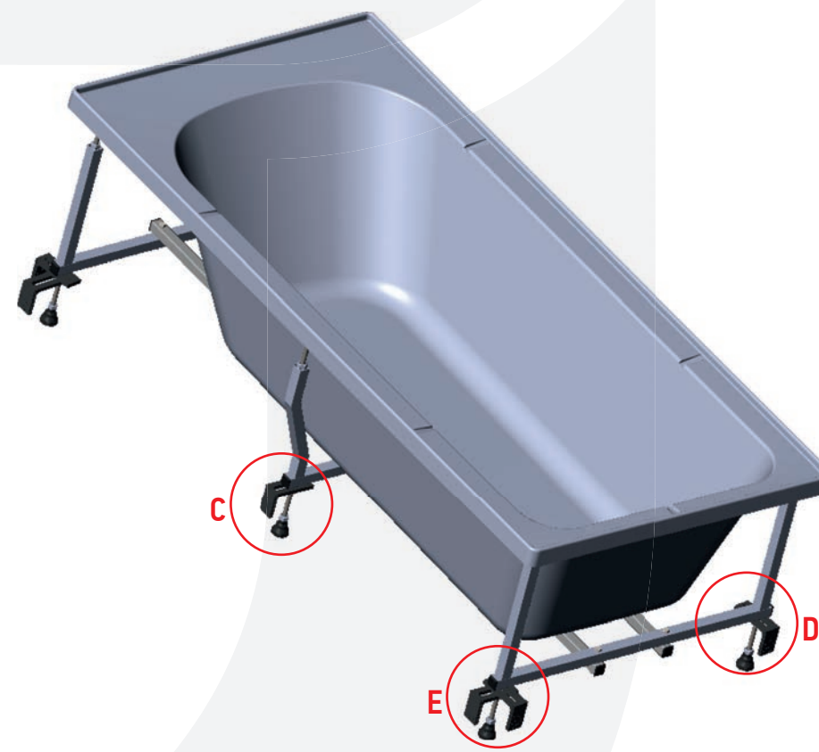
СБОРКА КАРКАСА ПОДДОНА БОКСОВ 1680x70
